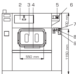
ВИД СПЕРЕДИ МВ 26 33 44
